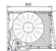
VEKAVARIANT 210 mm Revision vorne mit Insektenschutz
