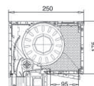
VEKAVARIANT 175 mm Revision unten mit Insektenschutz
